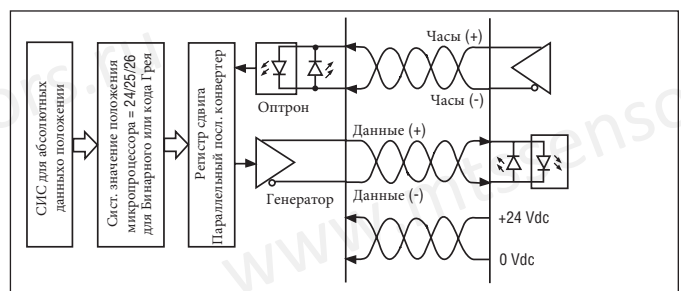
Рис. 11: Логическая диаграмма
