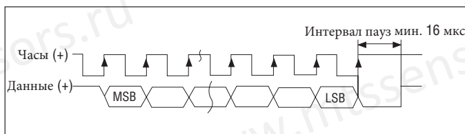
Рис. 9: Диаграмма времени
